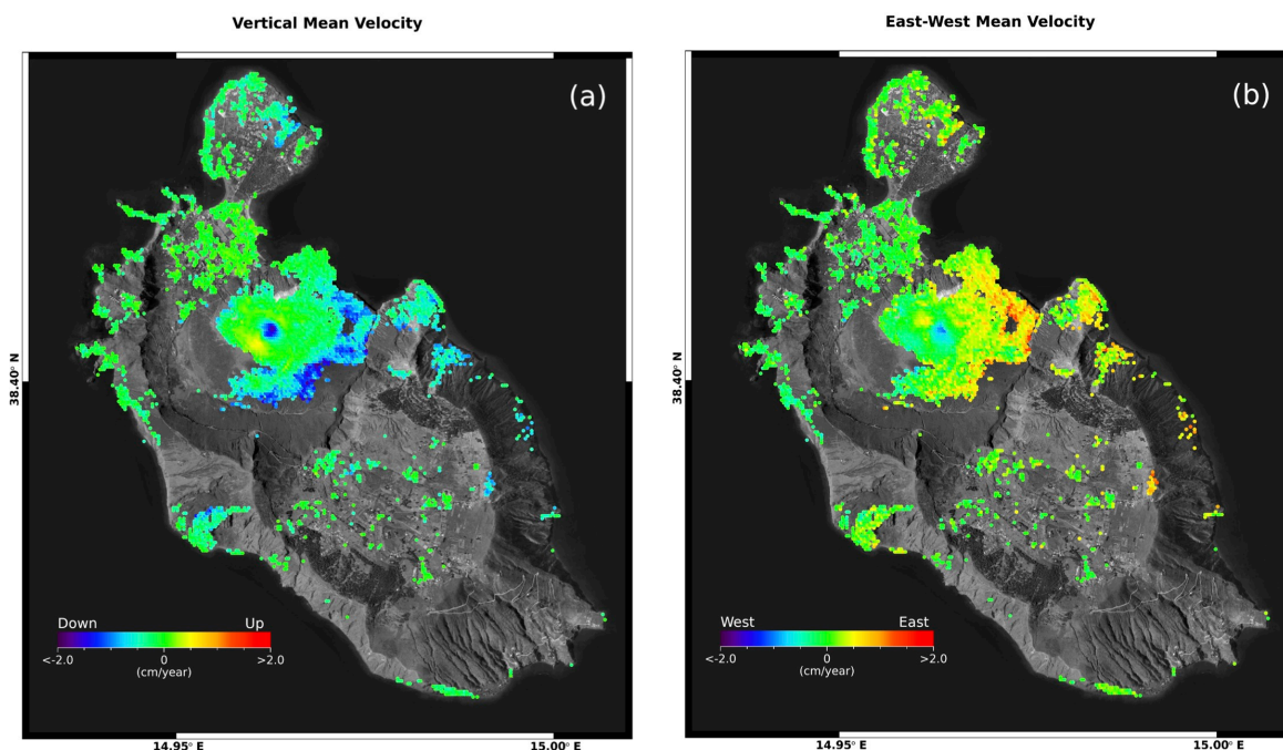
Figura 1. Vulcano: mappe delle componenti Verticale ed Est-Ovest della velocità media di deformazione relative al periodo 24 aprile 2015 – 5 febbraio 2023 generate a partire da dati Sentinel-1. a) Componente Verticale. b) Componente Est-Ovest.
