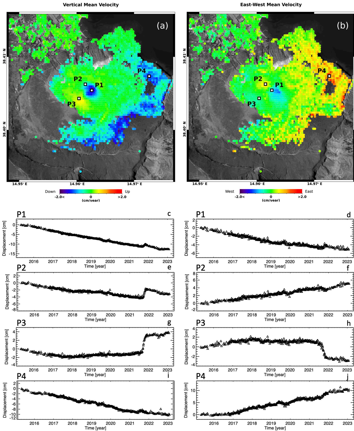
Figura 2. Vulcano – La Fossa: mappe delle componenti Verticale ed Est-Ovest della velocità media di deformazione relative al periodo 24 aprile 2015 – 5 febbraio 2023 generate a partire da dati Sentinel-1. a) Componente Verticale. b) Componente Est-Ovest. c-j) Andamento temporale della deformazione lungo la direzione Verticale (c)(e)(g)(i) ed Est-Ovest (d)(f)(h)(j) in corrispondenza di quattro punti identificati come P1, P2, P3 e P4 in (a)-(b).
