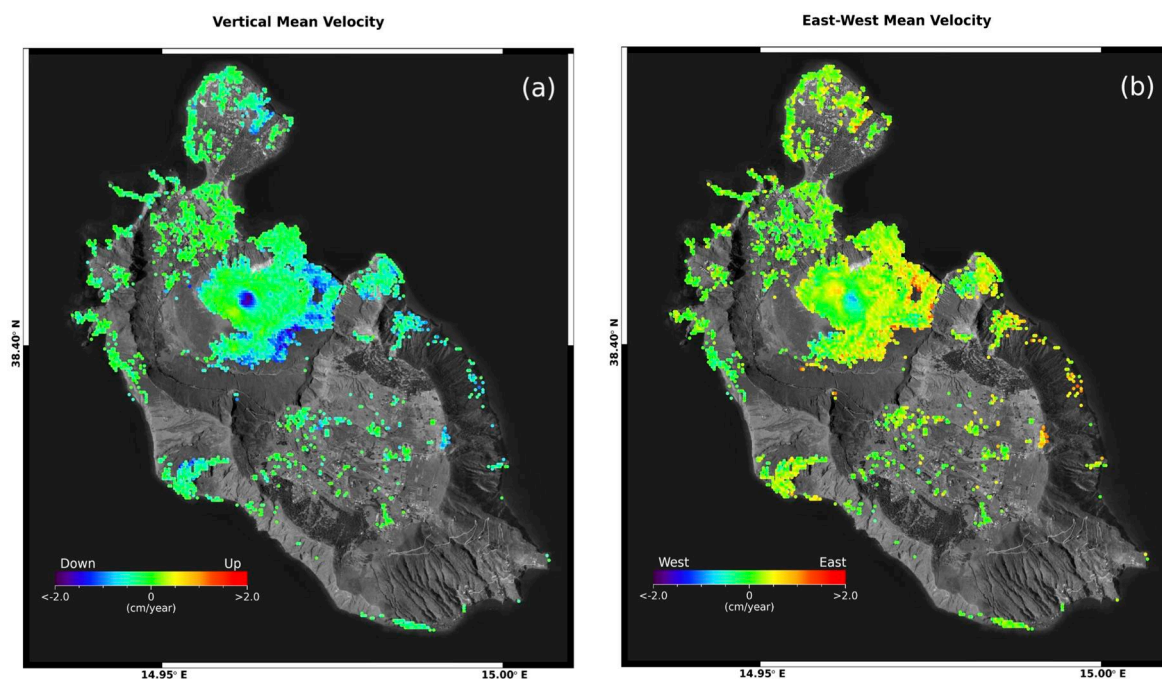
Figura 1. Vulcano: mappe delle componenti Verticale ed Est-Ovest della velocità media di deformazione relative al periodo 24 aprile 2015 – 4 luglio 2022 generate a partire da dati Sentinel-1. a) Componente Verticale. b) Componente Est-Ovest.
