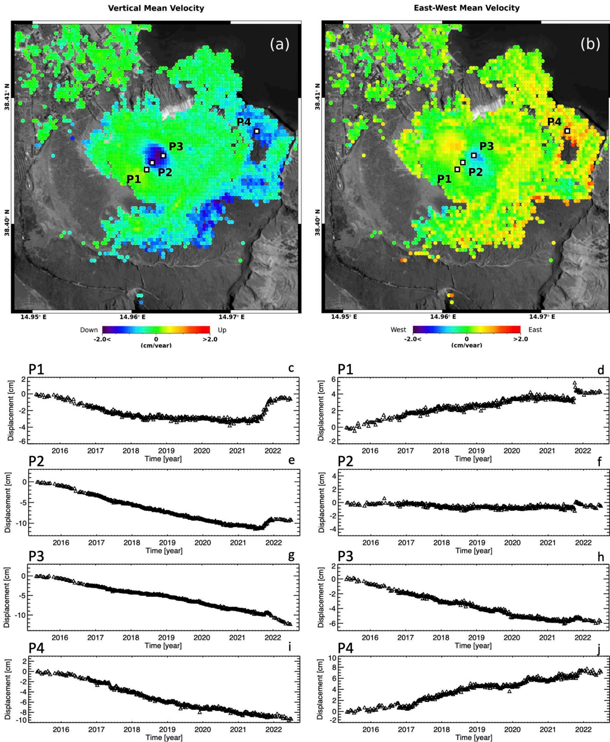
Figura 2. Vulcano – La Fossa: mappe delle componenti Verticale ed Est-Ovest della velocità media di deformazione relative al periodo 24 aprile 2015 – 4 luglio 2022 generate a partire da dati Sentinel-1. a) Componente Verticale. b) Componente Est-Ovest. c-j) Andamento temporale della deformazione lungo la direzione Verticale (c)(e)(g)(i) ed Est-Ovest (d)(f)(h)(j) in corrispondenza di quattro punti identificati come P1, P2, P3 e P4 in (a)-(b).
