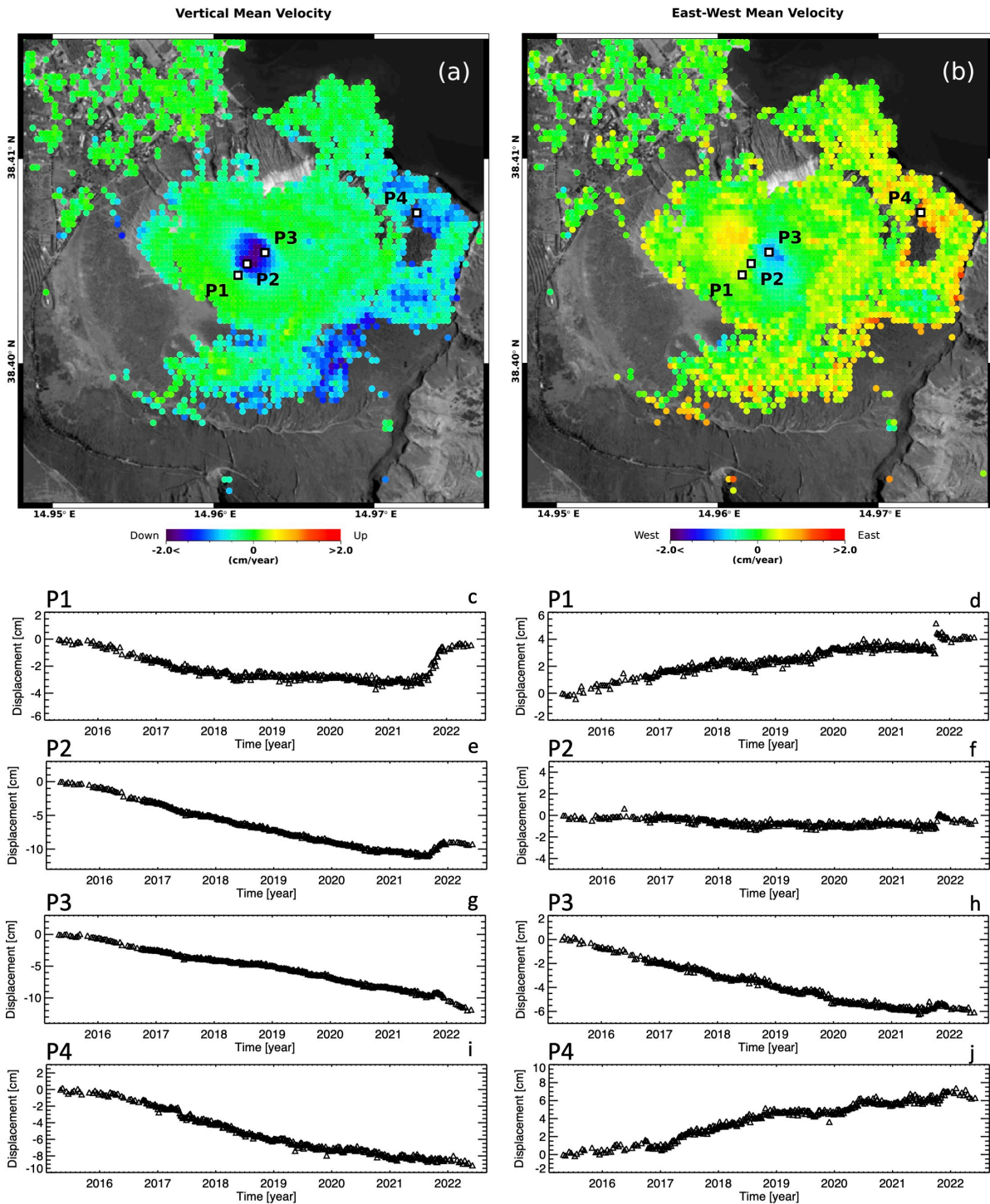
Figura 2. Vulcano – La Fossa: mappe delle componenti Verticale ed Est-Ovest della velocità media di deformazione relative al periodo 24 aprile 2015 – 10 giugno 2022 generate a partire da dati Sentinel-1. a) Componente Verticale. b) Componente Est-Ovest. c-j) Andamento temporale della deformazione lungo la direzione Verticale (c)(e)(g)(i) ed Est-Ovest (d)(f)(h)(j) in corrispondenza di quattro punti identificati come P1, P2, P3 e P4 in (a)-(b).
