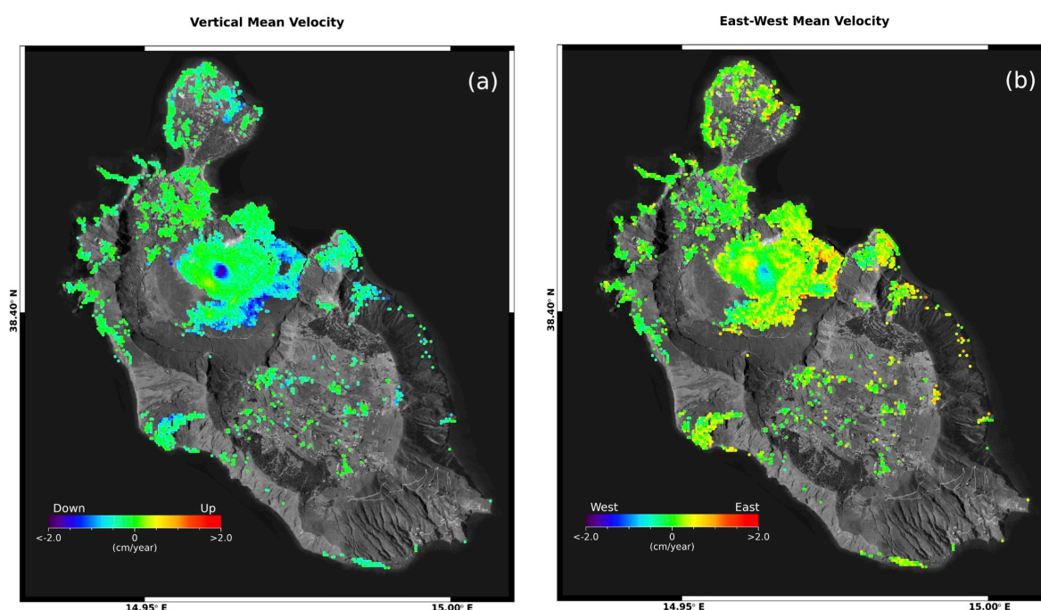
Figura 1. Vulcano: mappe delle componenti Verticale ed Est-Ovest della velocità media di deformazione relative al periodo 24 aprile 2015 – 10 giugno 2022 generate a partire da dati Sentinel-1. a) Componente Verticale. b) Componente Est-Ovest.
