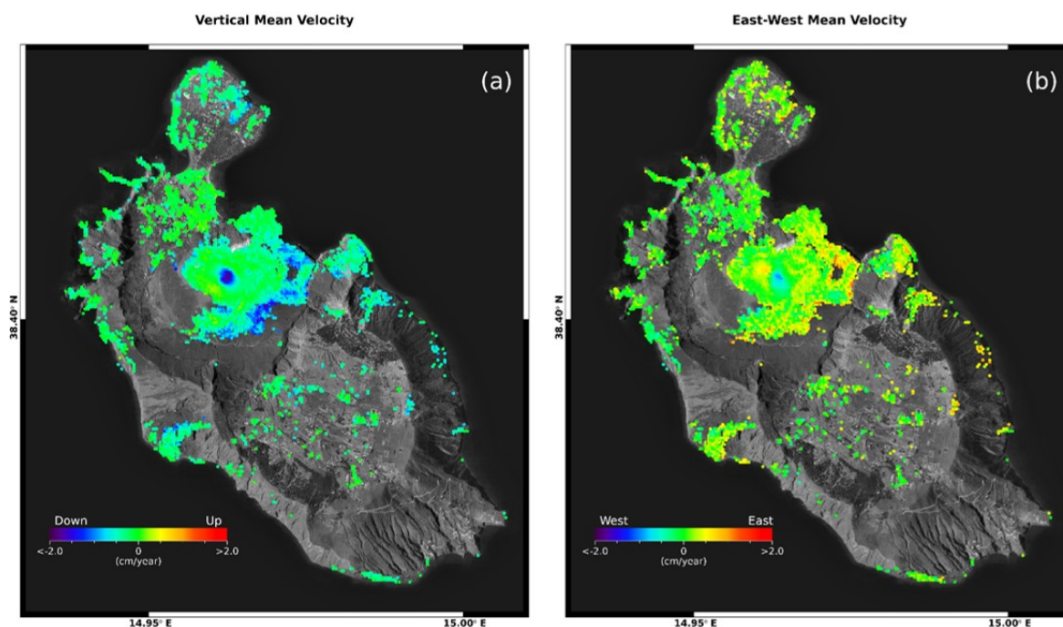
Figura 1. Vulcano: mappe delle componenti Verticale ed Est-Ovest della velocità media di deformazione relative al periodo 24 aprile 2015 – 6 marzo 2022 generate a partire da dati Sentinel-1. a) Componente Verticale. b) Componente Est-Ovest.
