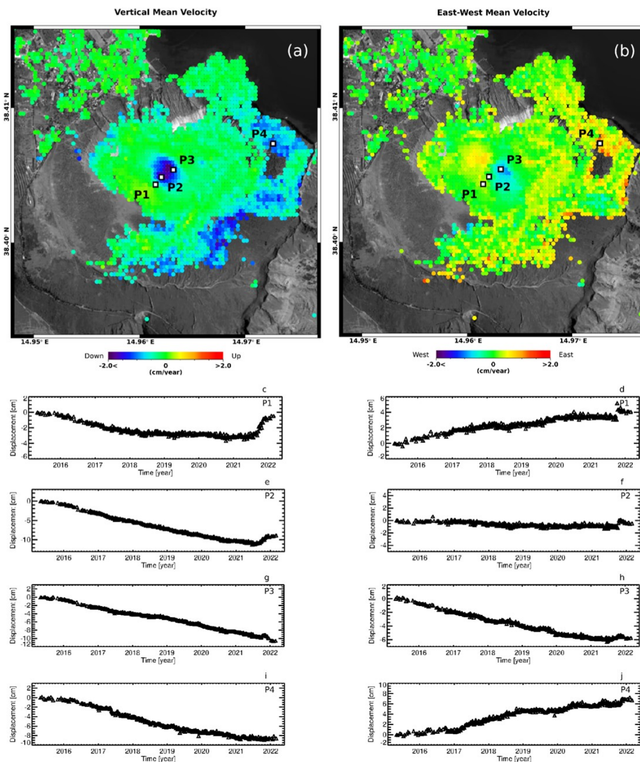
Figura 2. Vulcano – La Fossa: mappe delle componenti Verticale ed Est-Ovest della velocità media di deformazione relative al periodo 24 aprile 2015 – 6 marzo 2022 generate a partire da dati Sentinel-1. a) Componente Verticale. b) Componente Est-Ovest. c-j) Andamento temporale della deformazione lungo la direzione Verticale (c)(e)(g)(i) ed Est-Ovest (d)(f)(h)(j) in corrispondenza di quattro punti identificati come P1, P2, P3 e P4 in (a)-(b).
